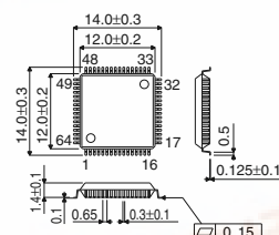
SQFP-T64
