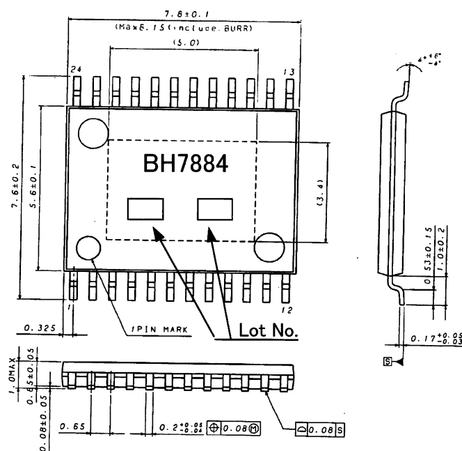
HTSSOP-B24 (Unit:mm)
