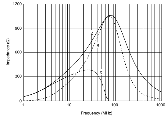
BLM21AH102SN1
