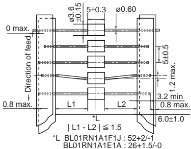
BL01RN
