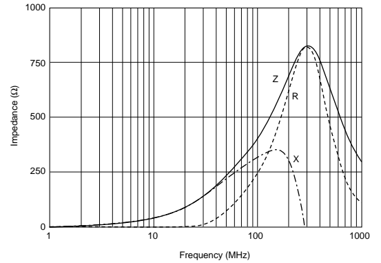
BLM18BD421SN1
