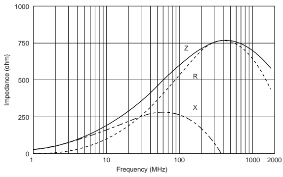
BLM18EG601SN1
