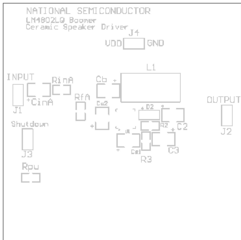
Top Overlay
