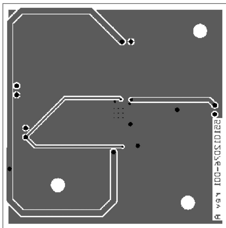
Bottom Layer
