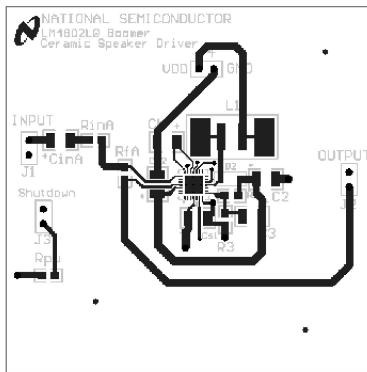
Top Layer
