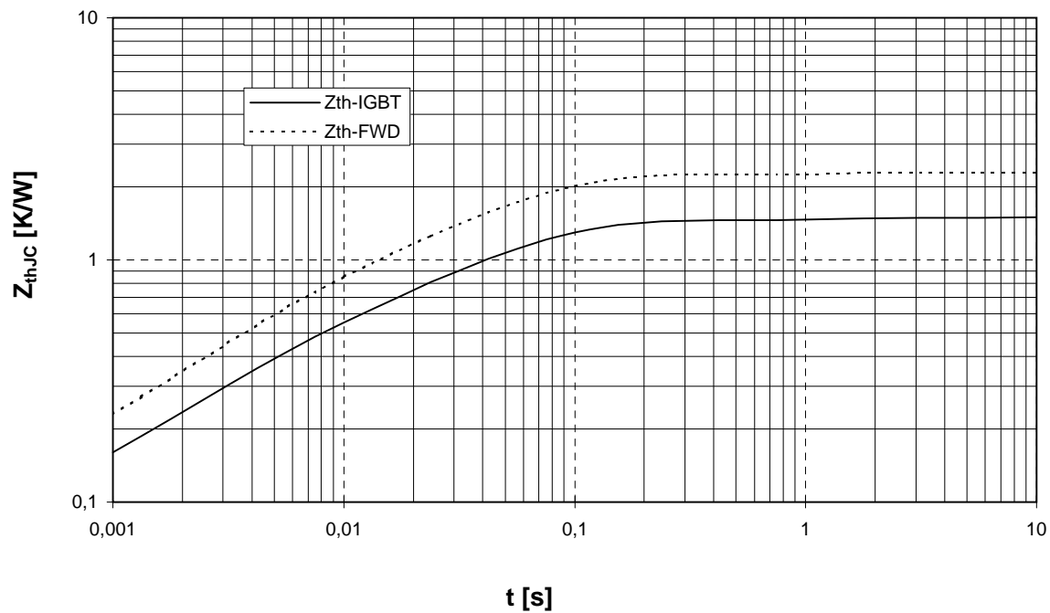
Transienter Wärmewiderstand Wechsler. Transient thermal impedance Inverter
