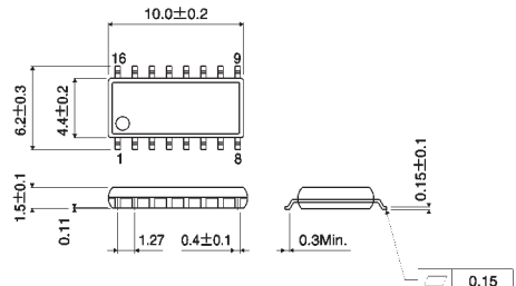
SOP16
