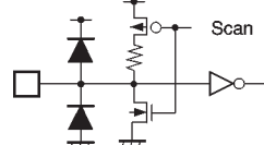
Keypad input
