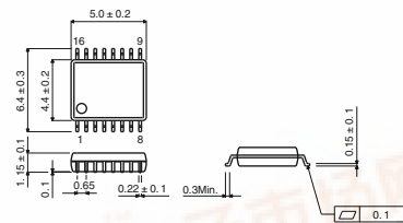
SSOP-B16
