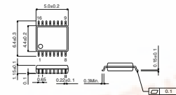
SSOP-B16
