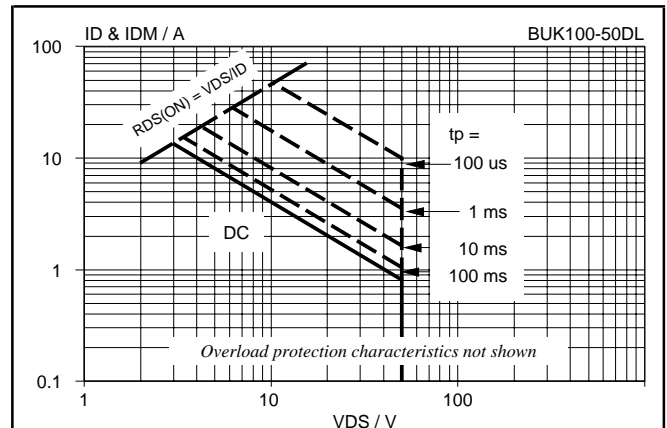
Fig.4. Safe operating area. T_{mb} = 25^\circ C I_D & I_{DM} = f(V_{DS}) ; I_{DM} single pulse; parameter t_p
