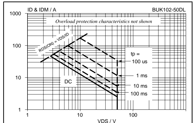
Fig.4. Safe operating area. T_{mb} = 25^\circ C I_D \text{ \& \ } I_{DM} = f(V_{DS}) ; I_{DM} single pulse; parameter t_p
