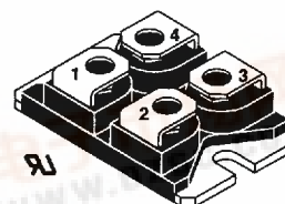
SOT-227B
