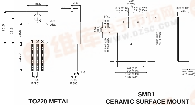
TO220 METAL
