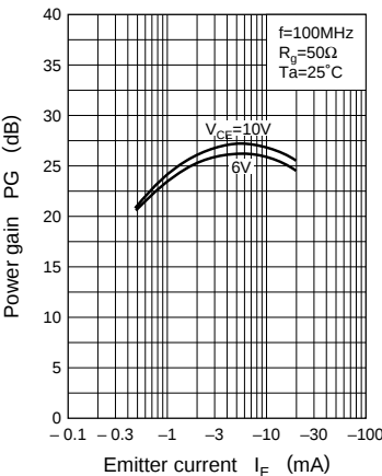
PG — I_E
