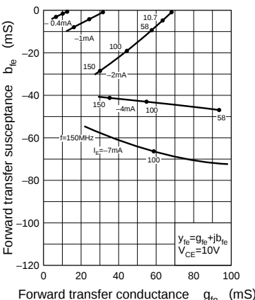
b_{fe} — g_{fe}
