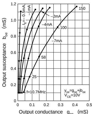
b_{oe} — g_{oe}
