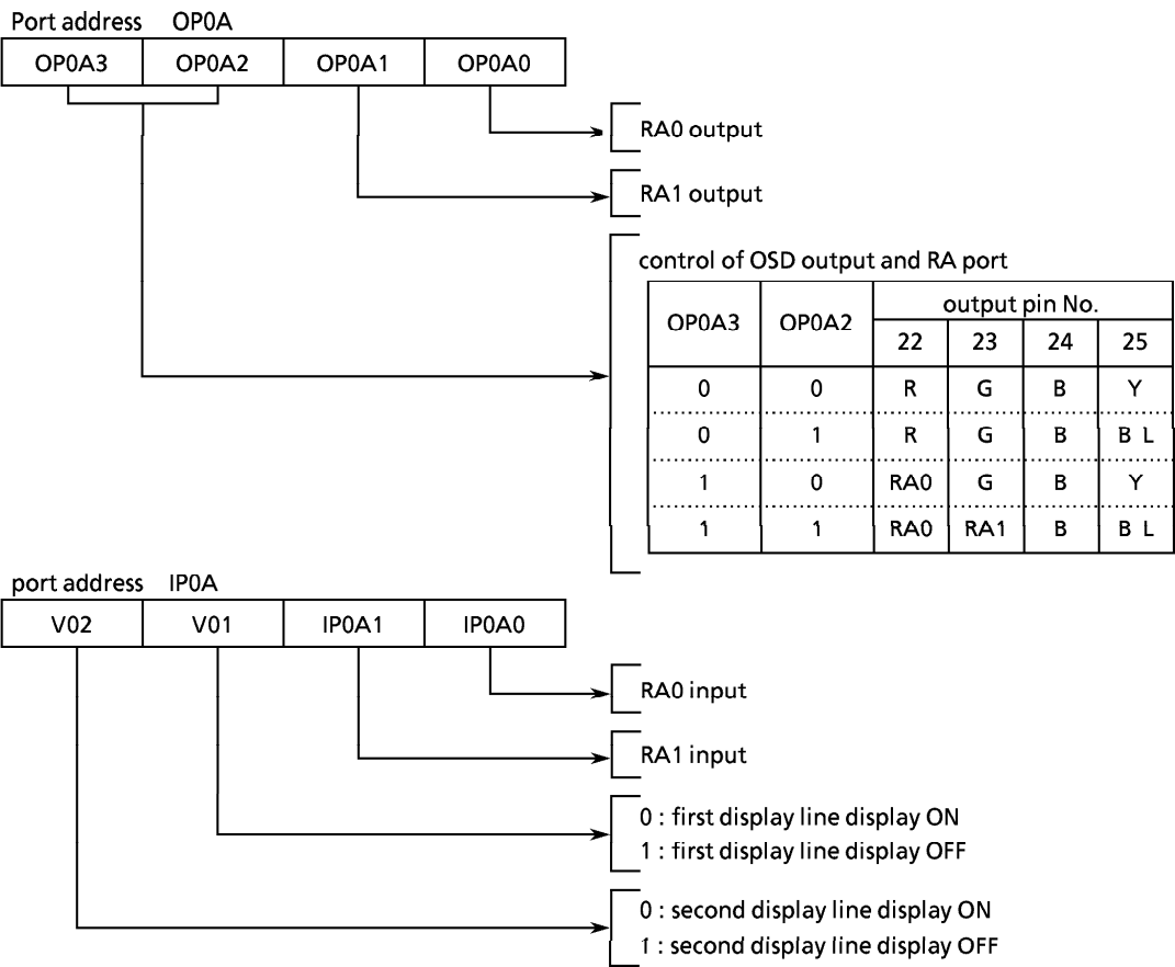
Figure 3-8. Port RA
