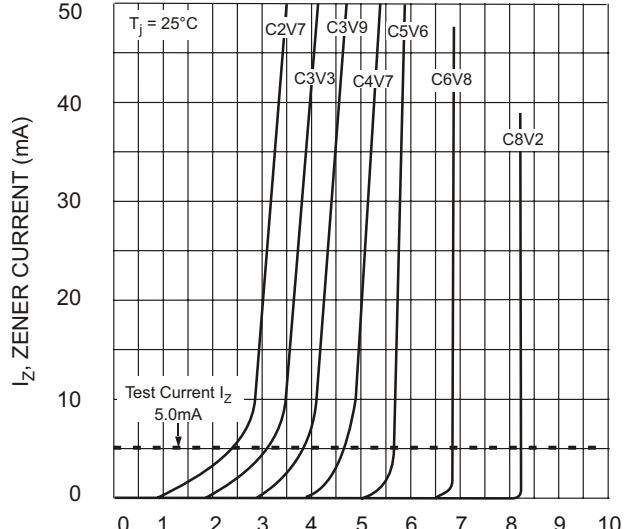
I_Z , ZENER CURRENT (mA) V_Z , ZENER VOLTAGE (V) Fig. 2. Zener Breakdown Characteristics
