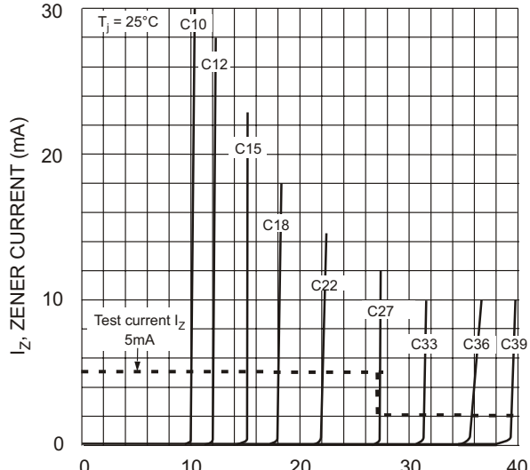
I_Z , ZENER CURRENT (mA) V_Z , ZENER VOLTAGE (V) Fig. 3. Zener Breakdown Characteristics
