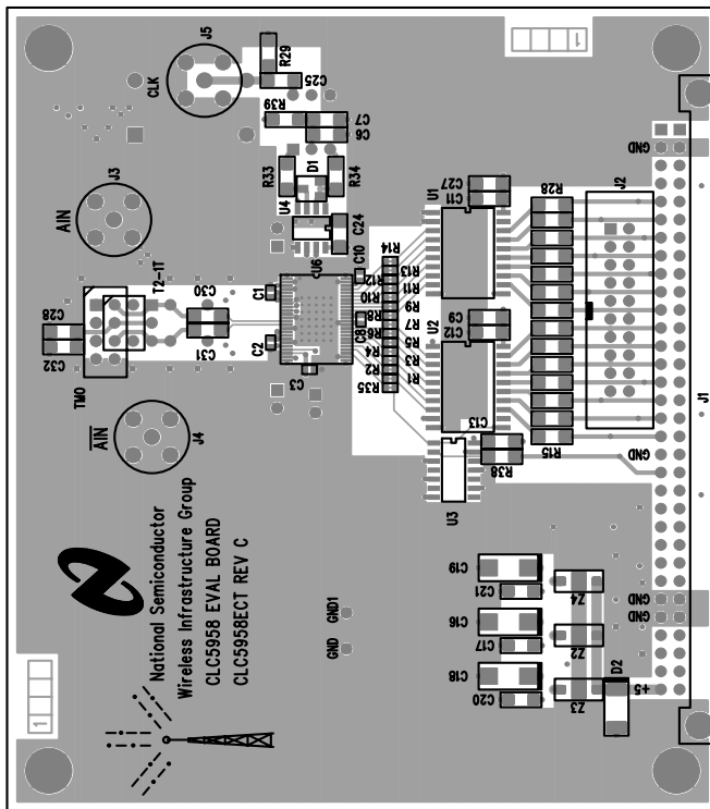
CLC5958PCASM Layer 1
