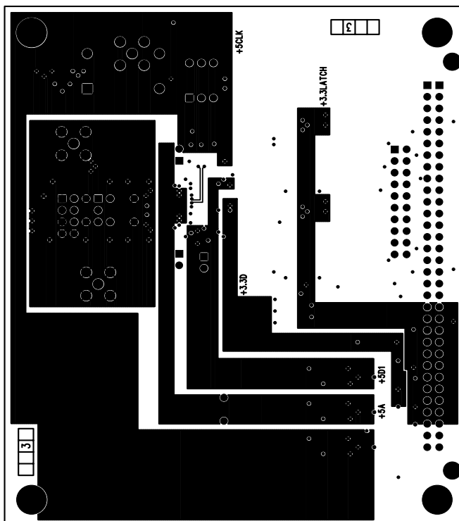
CLC5958PCASM Layer 3
