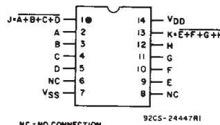
CD4002B
