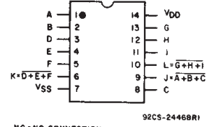
CD4025B
