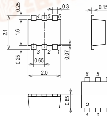
外形図 2173A (unit : mm)
