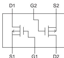
電氣的接続図
