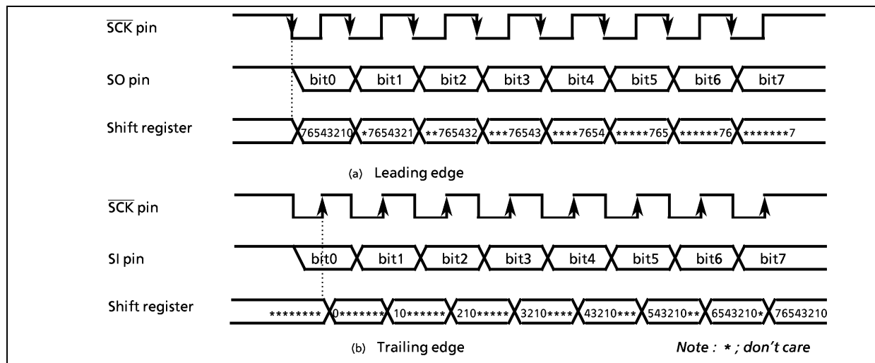
Figure 2-40. Shift Edge
