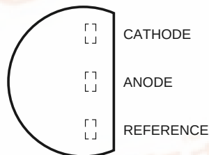
TO-92 (LP)
