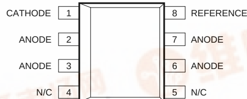
SOIC (D)
