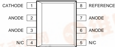
SOIC (D)
