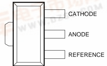
SOT-89 (S)
