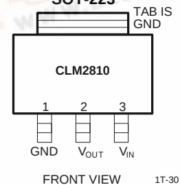
SOT-223
