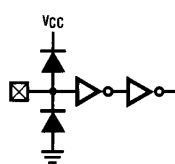
h. Hi-Z Input
