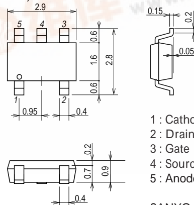
外形図 2171
