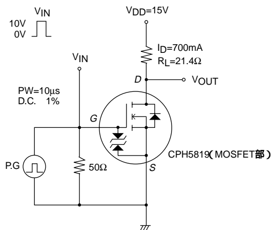
スイッチングタイム測定回路図 (MOSFET 部)
