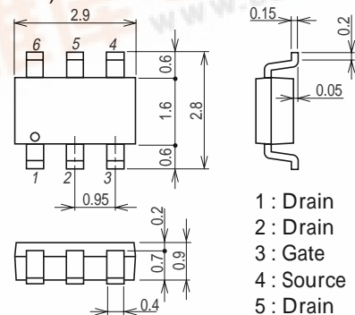
外形図 2151A
