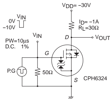
スイッチングタイム測定回路図
