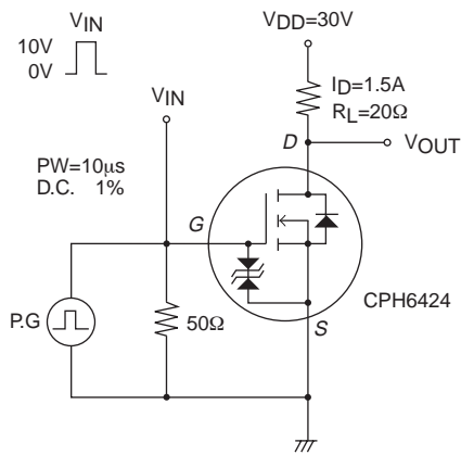
スイッチングタイム測定回路図
