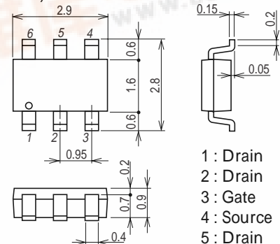
外形図 2151A
