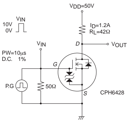
スイッチングタイム測定回路図
