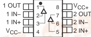
THS3122 SOIC (D) AND SOIC PowerPAD™ (DDA) PACKAGE (TOP VIEW)
