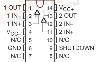
THS3125 SOIC (D) AND TSSOP PowerPAD™ (PWP) PACKAGE (TOP VIEW)
