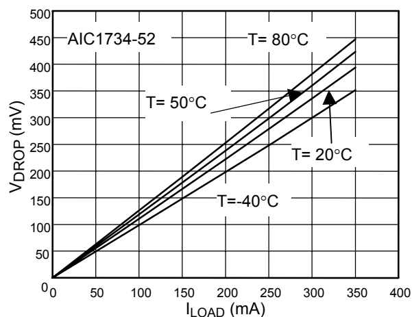
Fig. 7 V_{DROP} vs. I_{LOAD}
