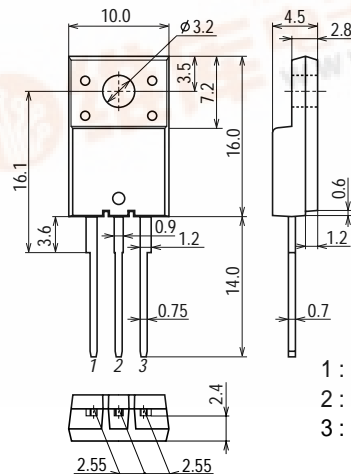
外形図 2079D (unit : mm)
