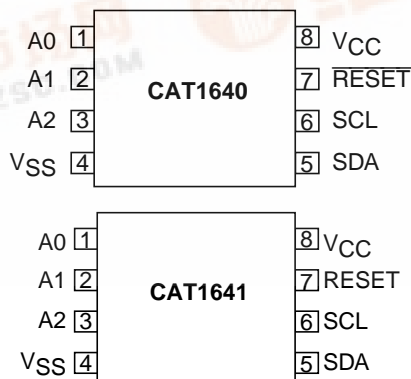
TSSOP (U, Y)
