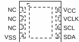
TDFN Package (RD4, ZD4)
