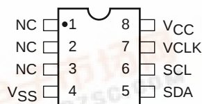
TDFN Package (RD4, ZD4)
