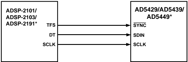
Figure 48. ADSP-2101/ADSP-2103/ADSP-2191 SPORT to AD5429/AD5439/AD5449 Interface
