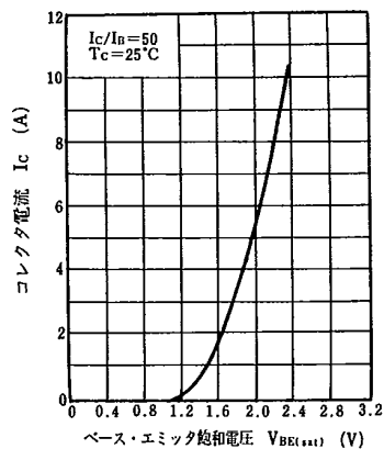
I_C - V_{BE(sat)}
