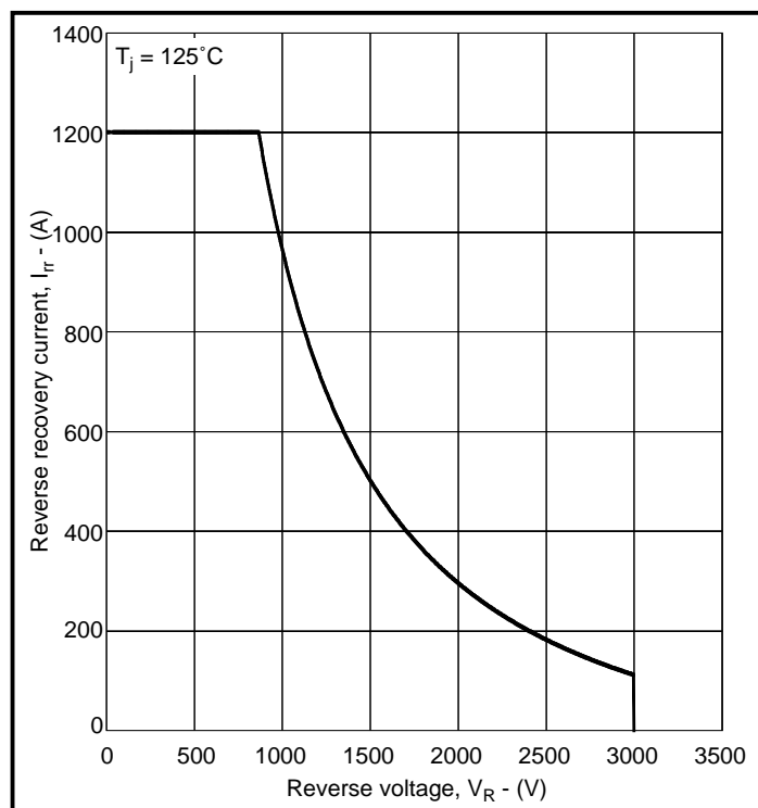
Fig. 7 RBSOA
