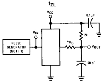
TL/F/7506-7
