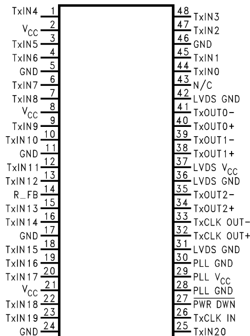
DS90C365AMT
