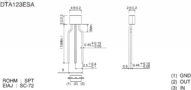
DTA123ESA
