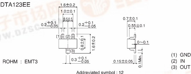
DTA123EUA
