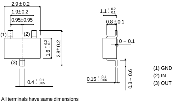
EIAJ: SC— 59
