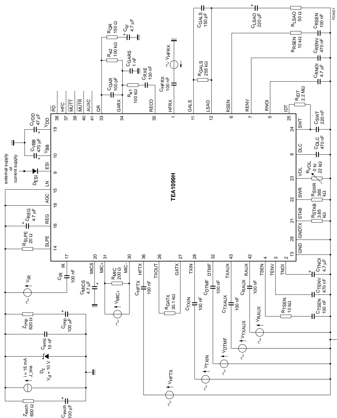
Fig.15 Test circuit.
