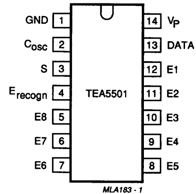
Fig.2 Pinning diagram.
