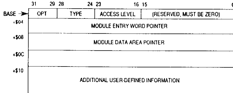
Figure 9-10. Module Descriptor Format
