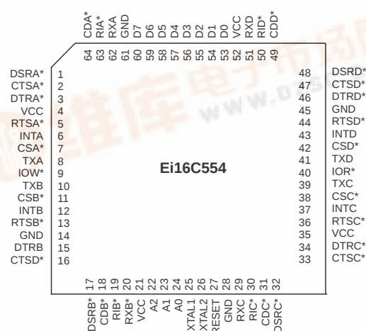
64-PIN TQFP
