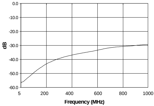
L-I Isolation
