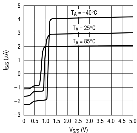
I_{S/S} vs V_{S/S}
