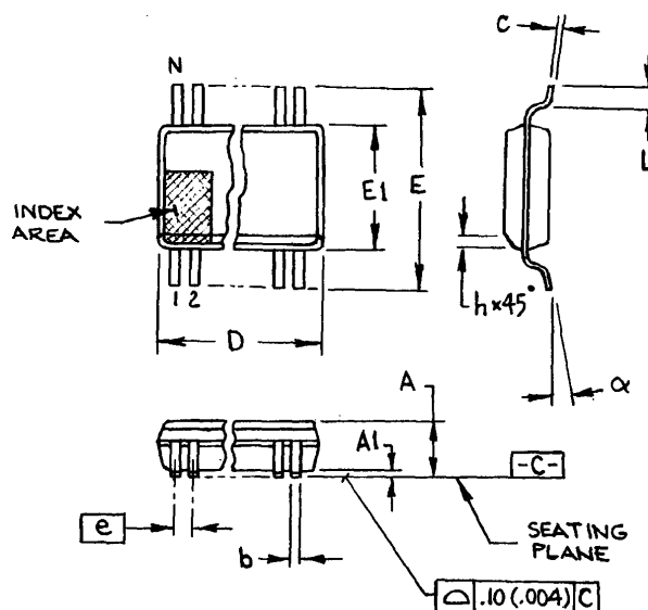
300 mil SSOP
