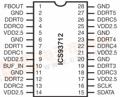
28-Pin SSOP
