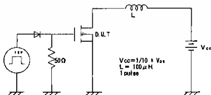
図1 測定回路
