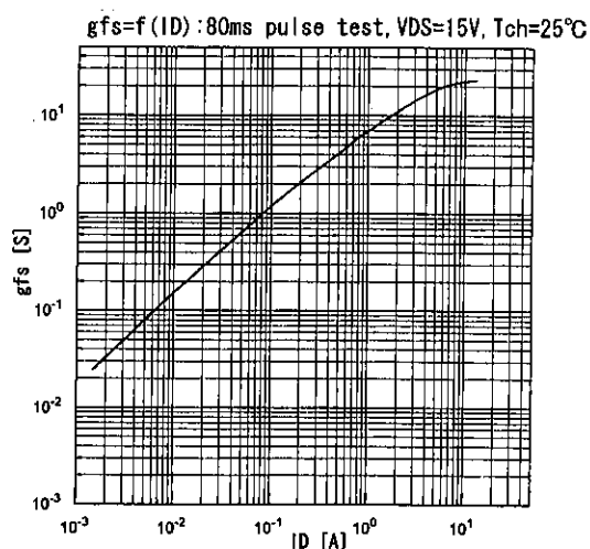
伝達コンダクタンス Typical transconductance
