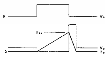
図2 動作波形
